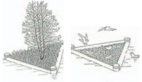
Element pływający z roślinnością typ SRD.
